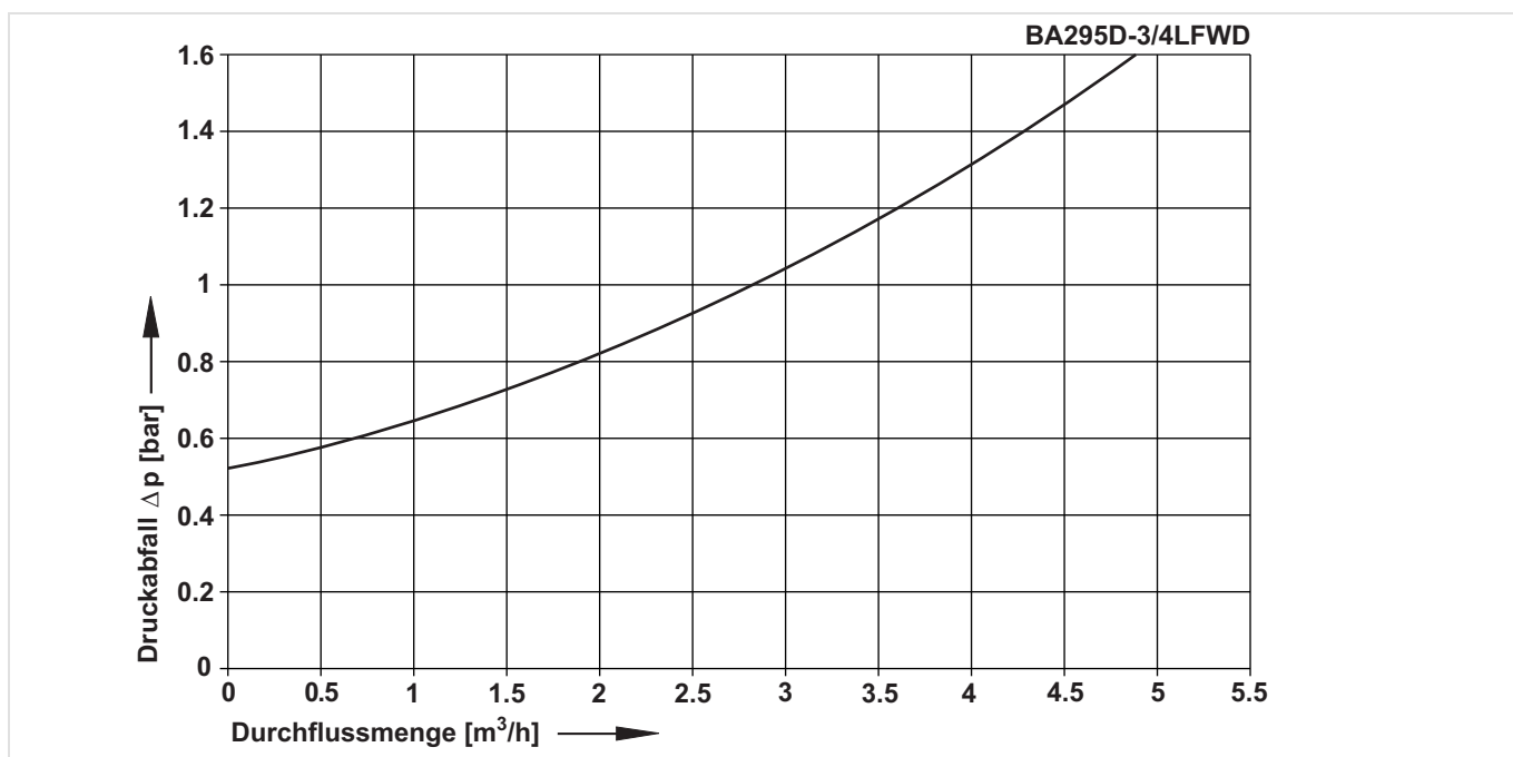
Abb. 2 Druckabfall innerhalb des Ventils abhängig vom Durchfluss
