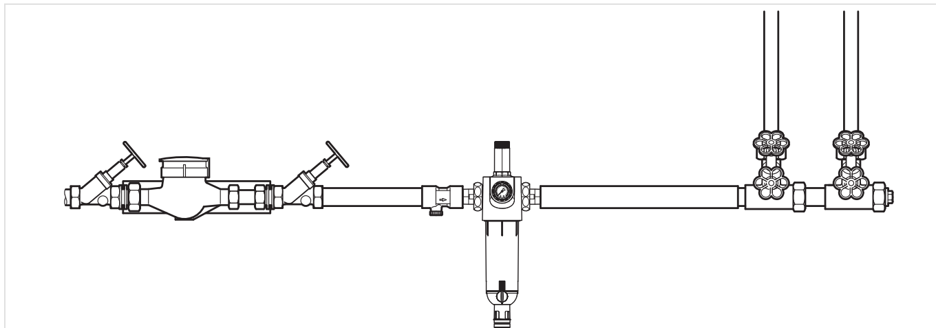
FK74CS-LF 1 1/2" - 2"
