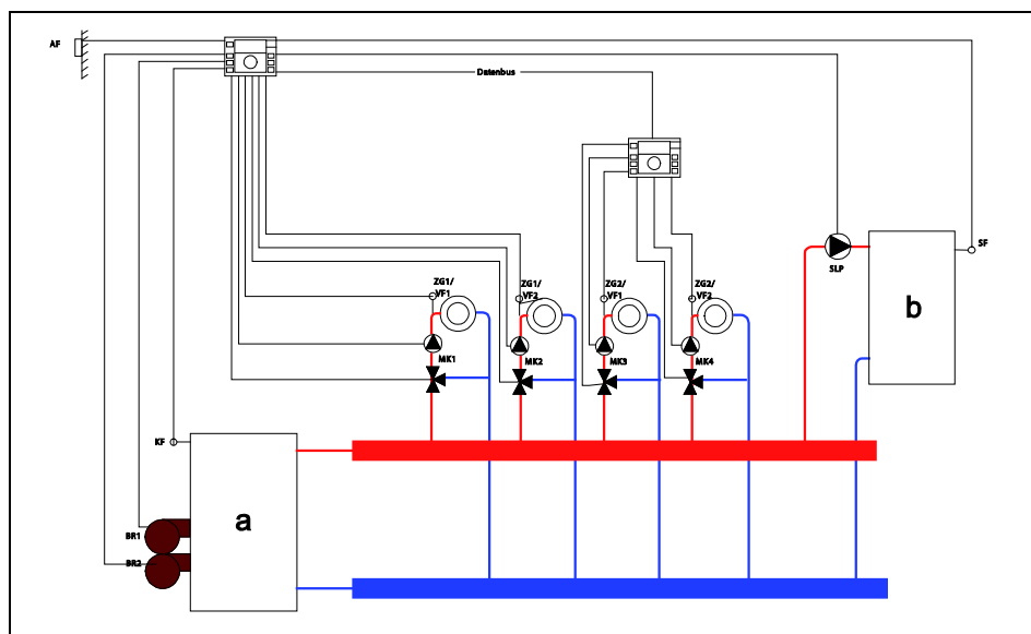
a Heizkessel
