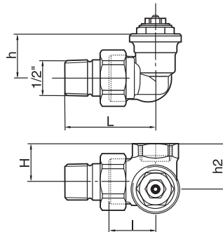
Fig. 9. Corner angle
