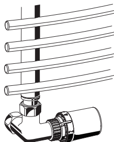
Fig. 6. Double angle (coin) gauche sur un radiateur sèche-serviettes
