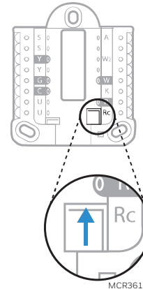
Onglet coulissant R/Rc
