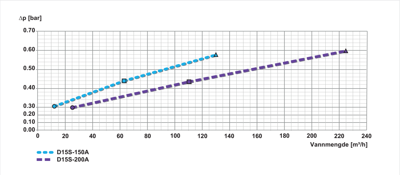
Fig. 3 Trykkfall inne i ventilen er avhengig av vannmengden og tilkoblingsdimensjonen som er brukt (dimensjon 150-200) Trykkinnstilling: P1: 8 bar, P2: 3 bar
