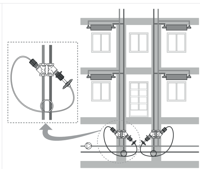
Rys. 2. Zastosowanie regulatora w instalacji chłodzenia
