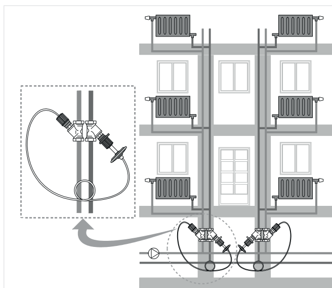
Rys. 1. Regulator membranowy Kombi-DP w instalacji ogrzewania
