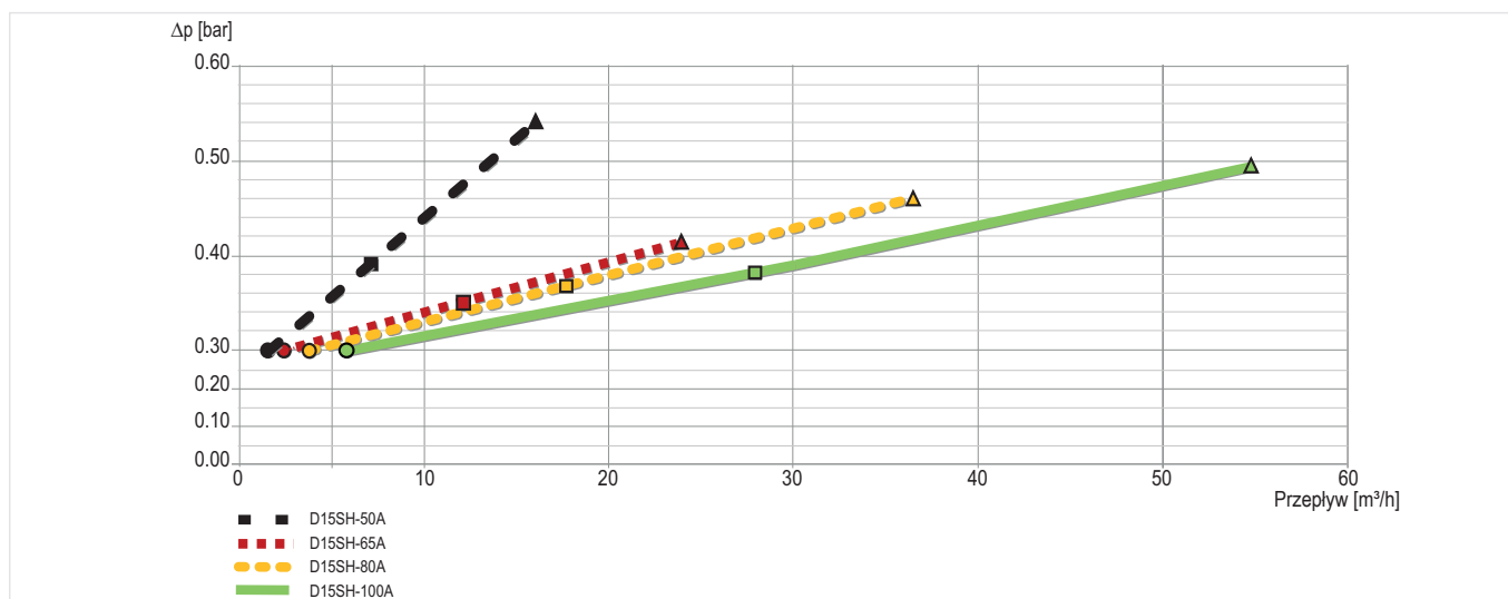
Rys. 2 Spadek ciśnienia na zaworze dla różnych średnic (DN 50 - dn100)
