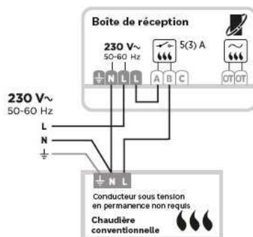
Chaudière conventionnelle 230 V
