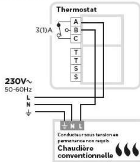
Chaudière conventionnelle 230 V
