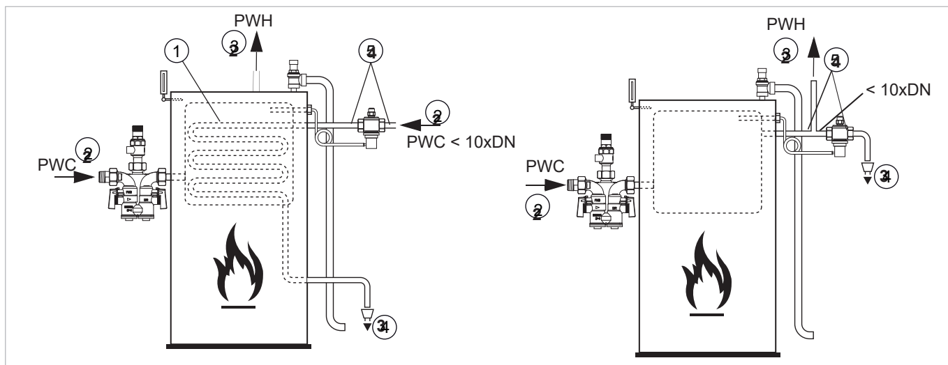
Obr. 1 příklady běžné instalace odpouštěcího ventilu
