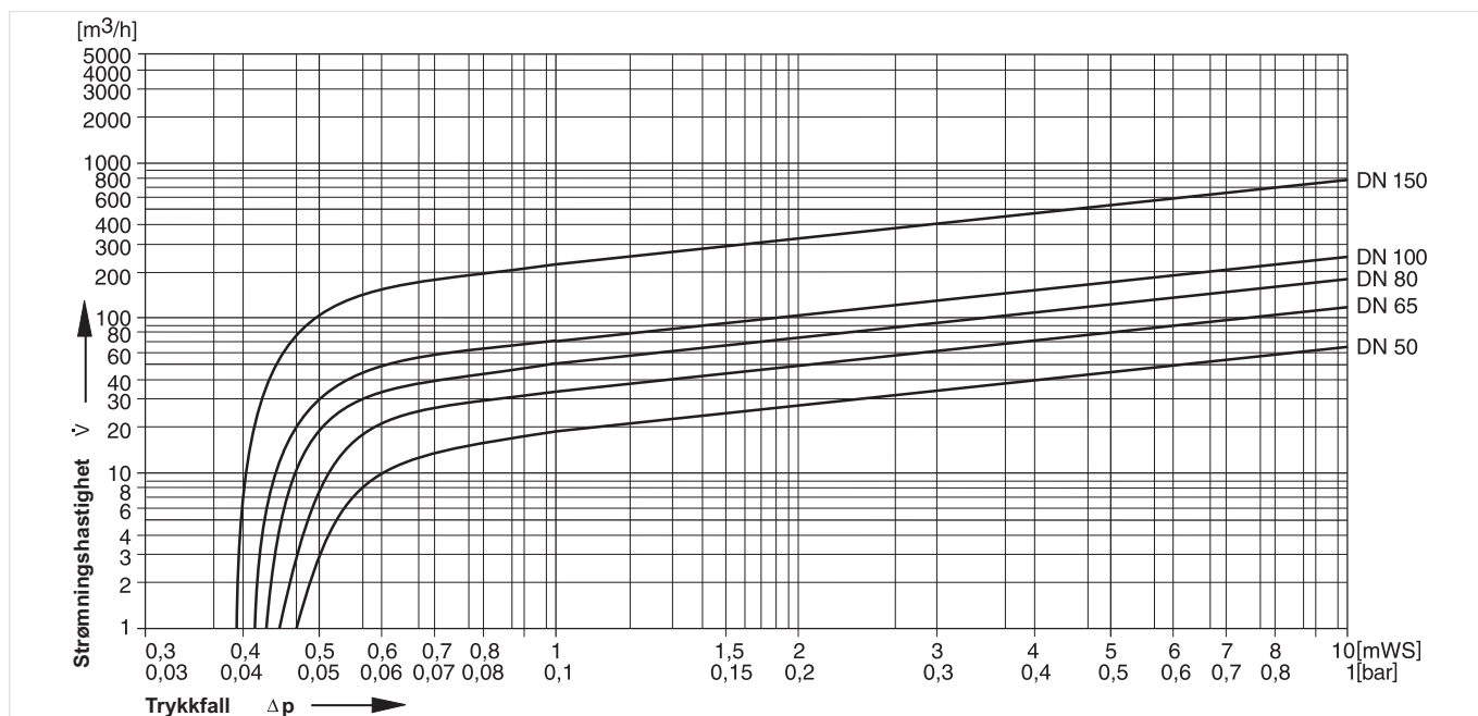
Fig. 1 Trykkløst fall inne i ventilen avhengig av vannmengden og tilkoblingsdimensjonen som er brukt
