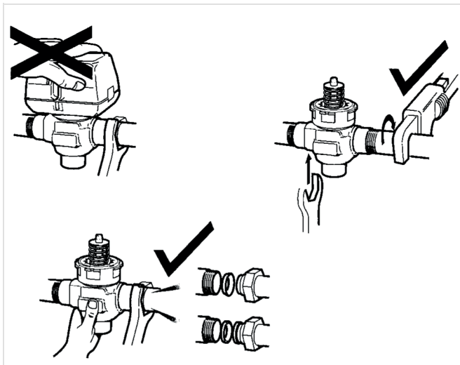
Abb. 5 Rohrleitungen
