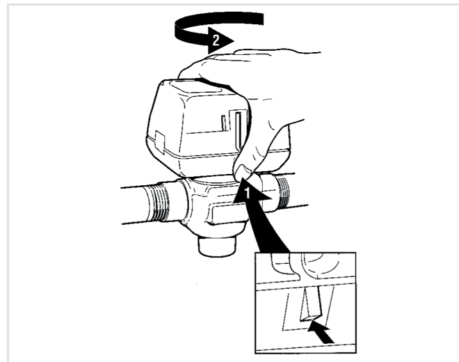
Abb. 6 Schnappverschluss
