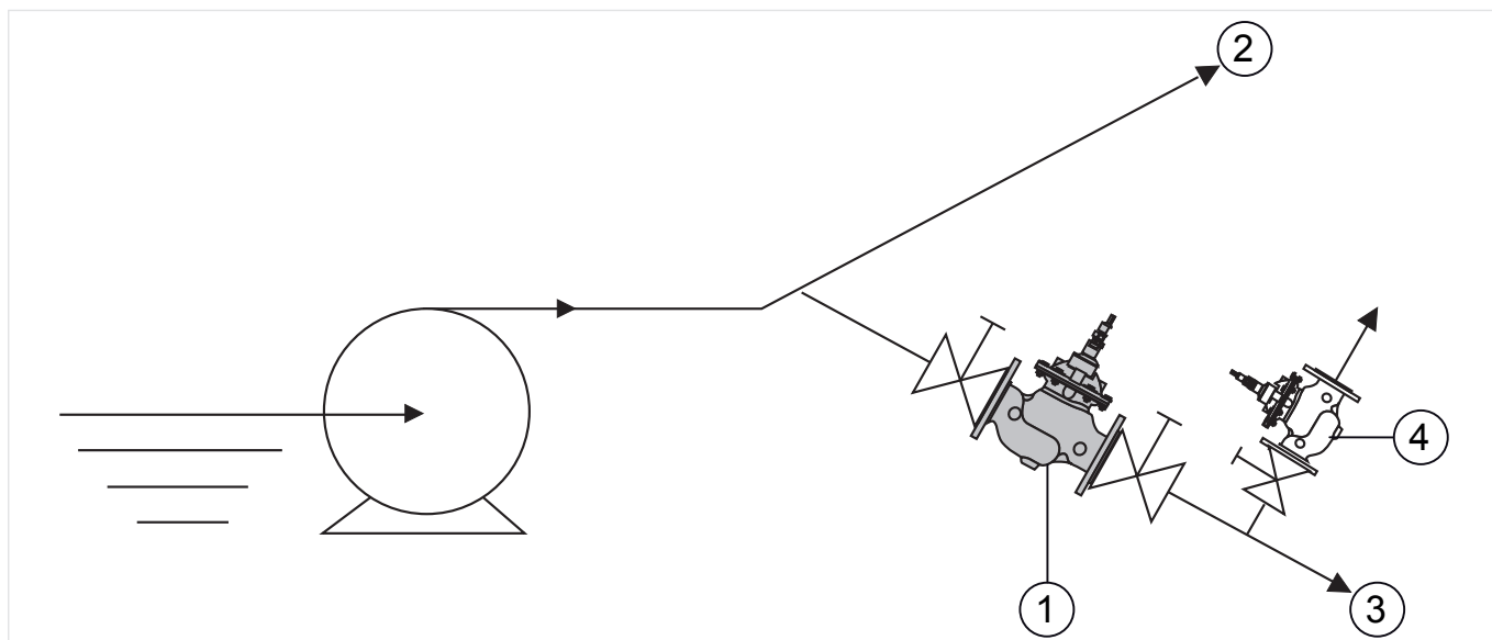
Fig. 1 Eksempel på standard installasjon av trykkreduksjonsventil
